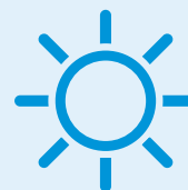
Standardnetze
